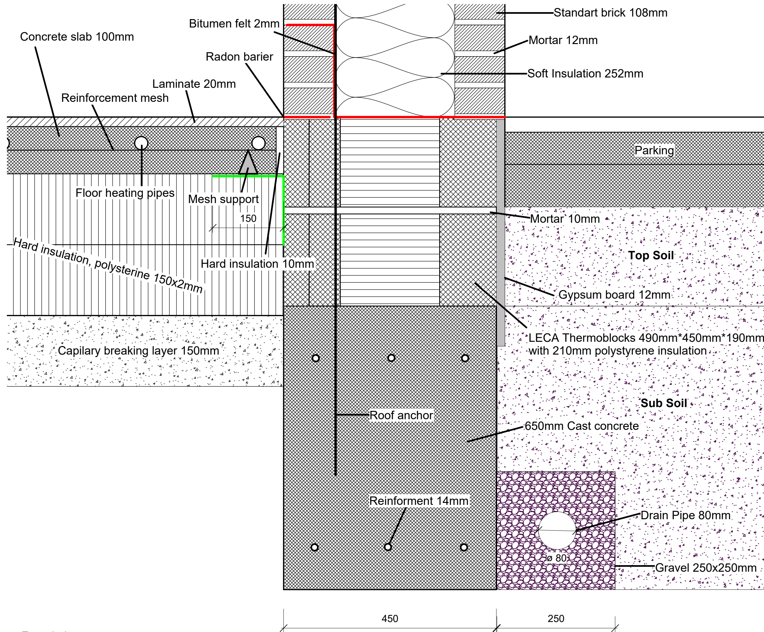
Foundation 1 : 5
